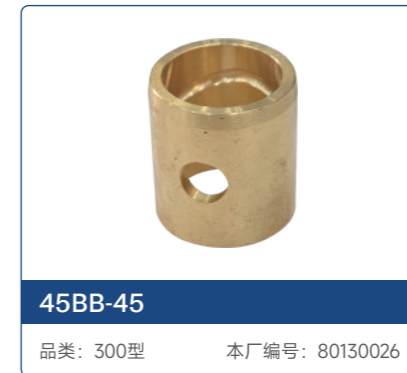
轴衬
